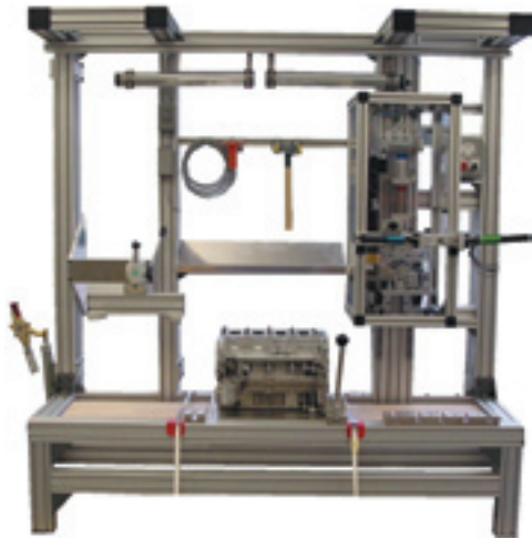
Montagearbeitsplatz für Motorenbau
