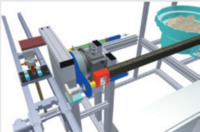
Bestückungsanlage für Elektromotoren
